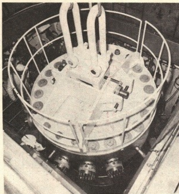
Embarquement de la cuve du réacteur.
