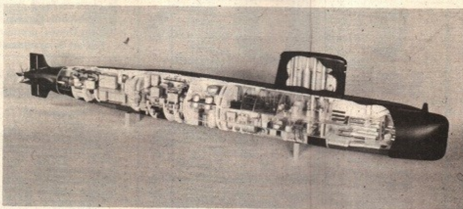
Coupe du sous-marin nucléaire d'attaque.
