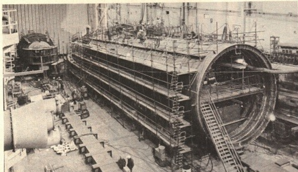
La coque en cours de construction.
