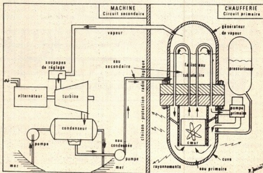
Schéma du réacteur.
