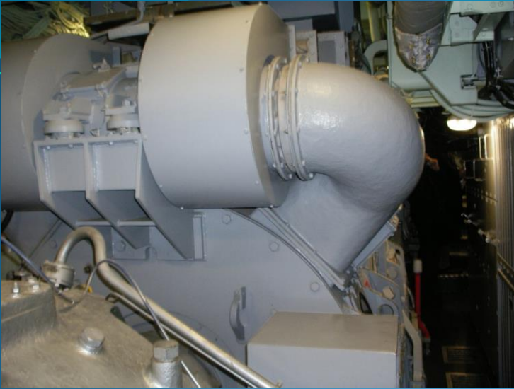
Moteur Electrique de propulsion
